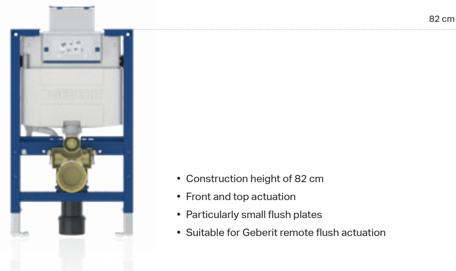
Geberit Omega concealed cistern
